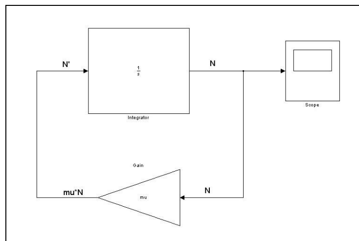
Abb. 3: Simulink-Modell zur numerischen Lösung von (0.4)
