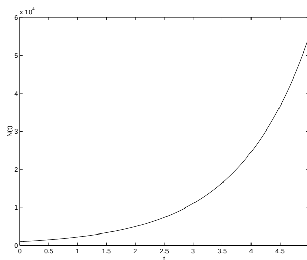
Abb. 2: Exakte Lösung zu (0.4) mit N(0) = 10^3 und \mu = 0.8
